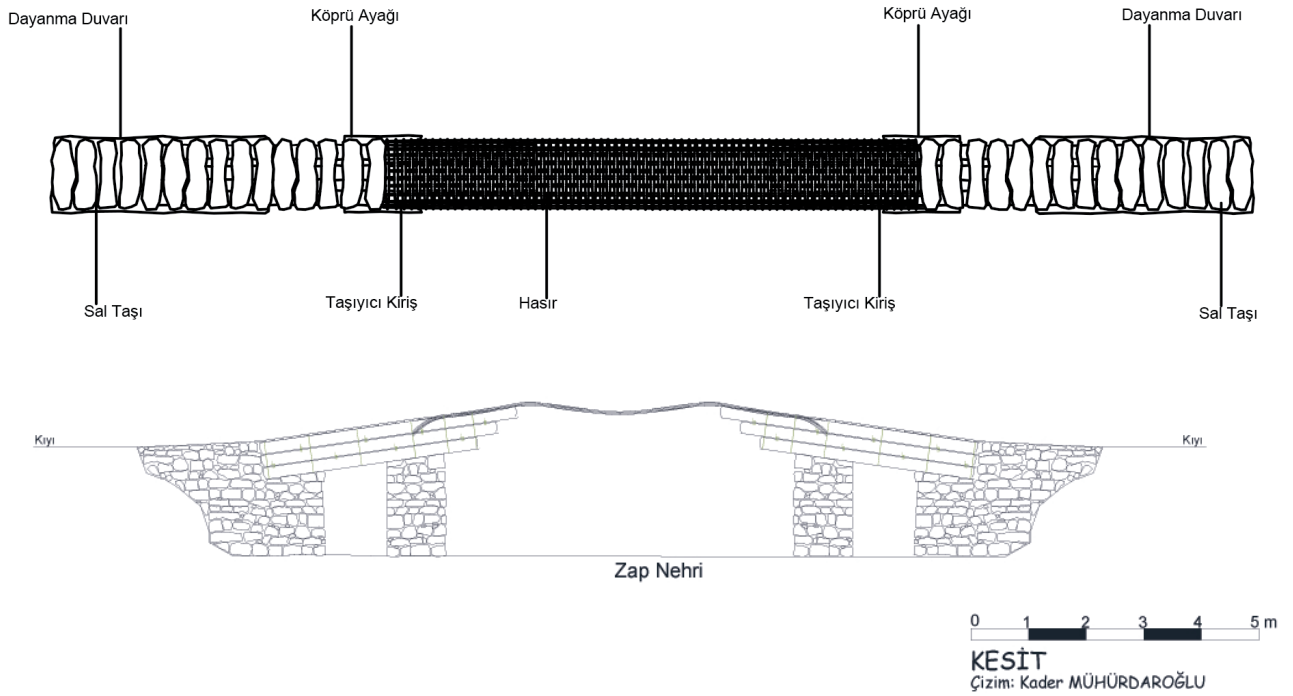
Resim 12. Hakkârî'nin tarihi ahşap hasır köprü planı (Çizim: Kader Mühürdaroglu).
